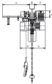
Motorfahwerk
