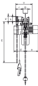
Haspelfahwerk
